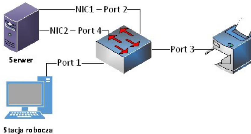
Rys. Schemat połączenia urządzeń sieciowych
